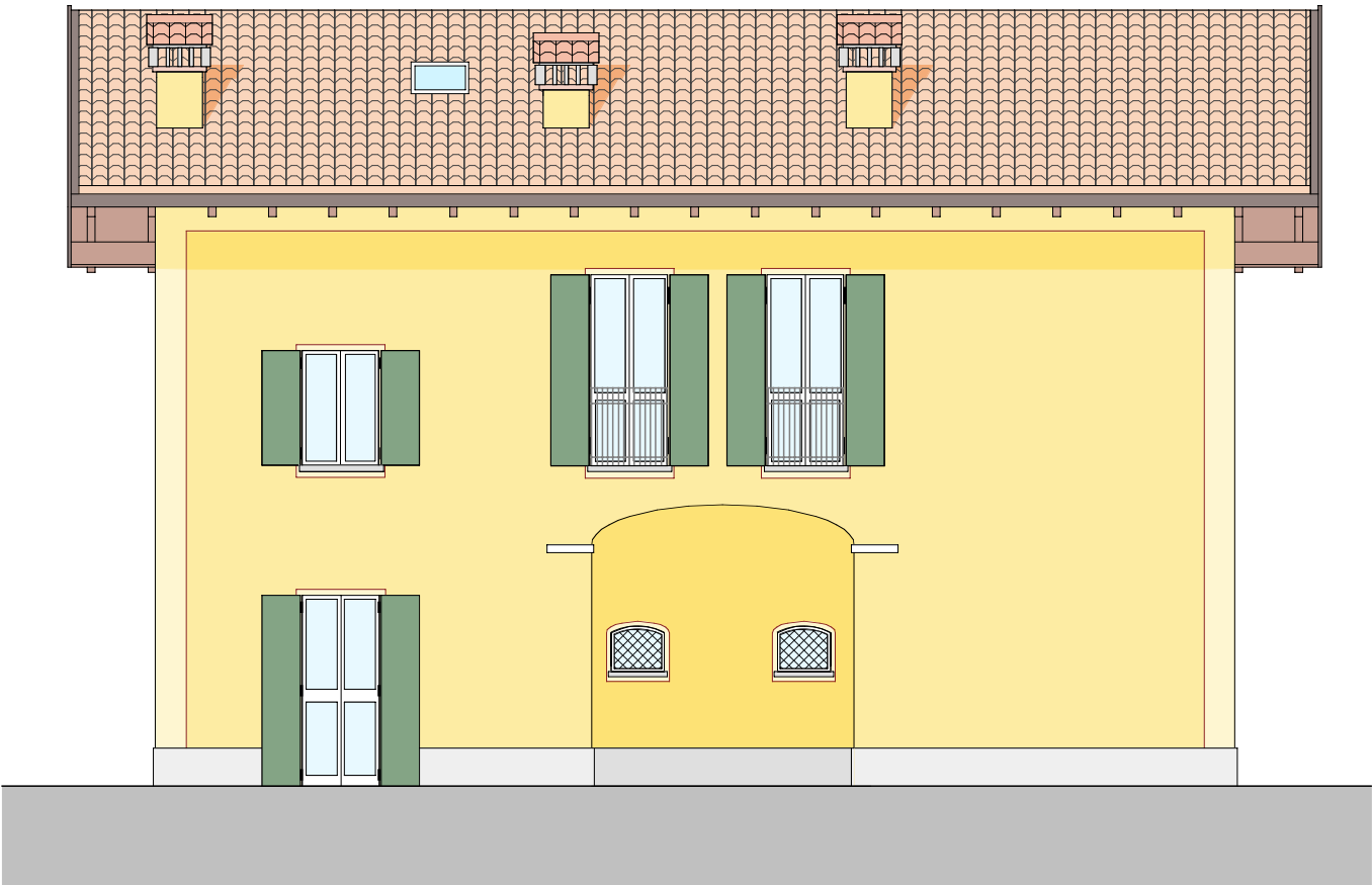
PROSPETTO SUD
