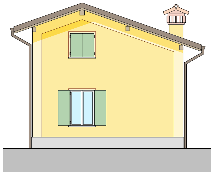
PROSPETTO OVEST
