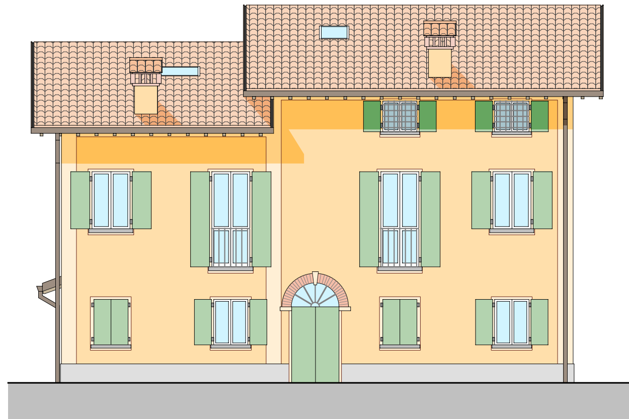
PROSPETTO SUD
