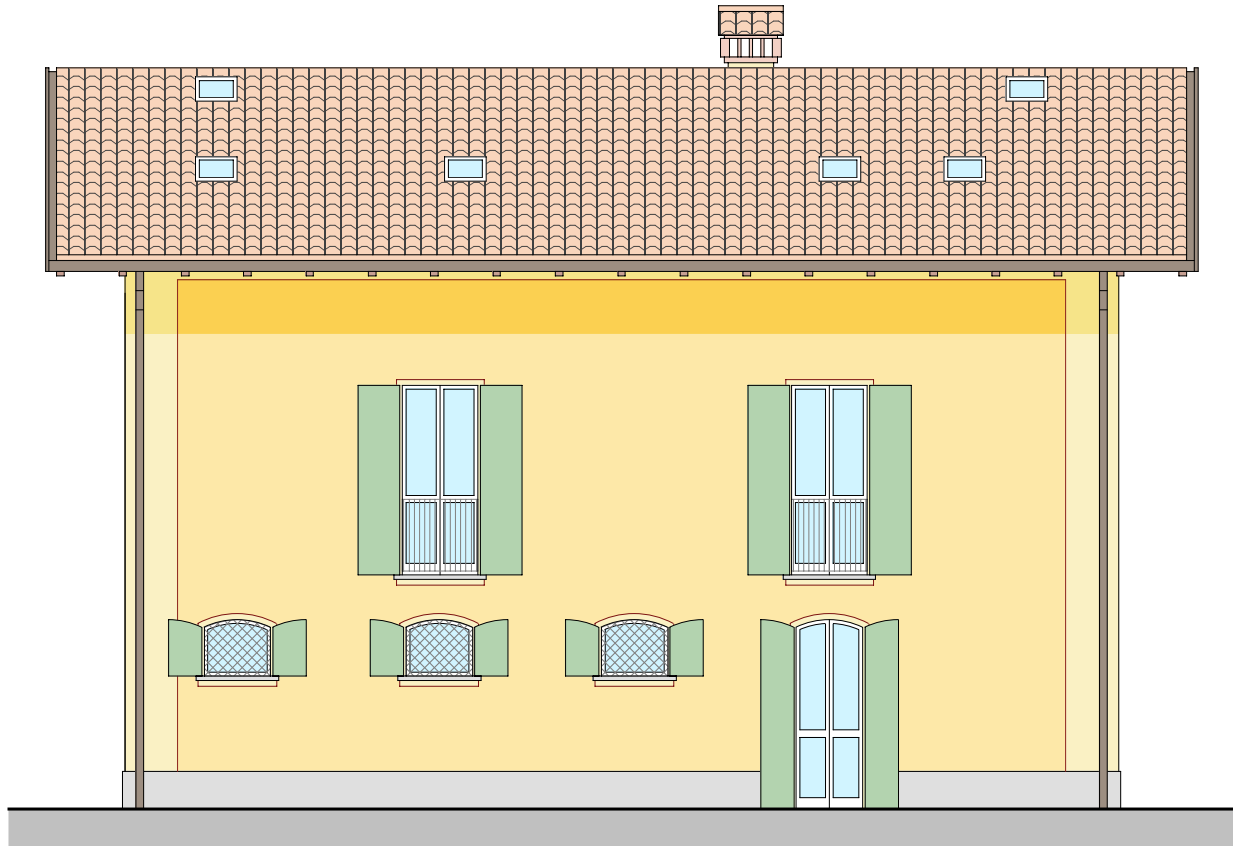
PROSPETTO NORD
