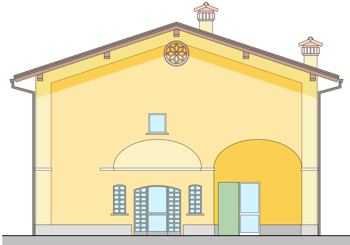
PROSPETTO SUD
