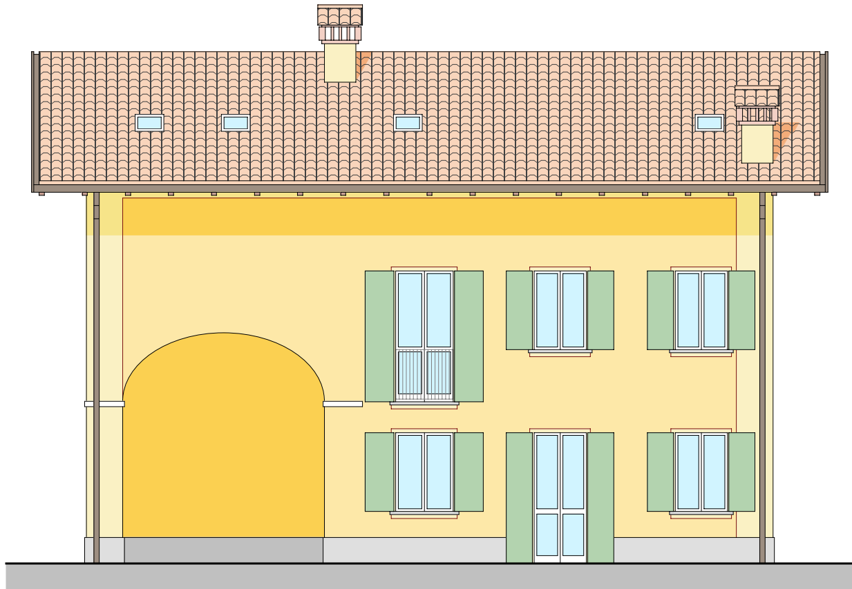
PROSPETTO SUD
