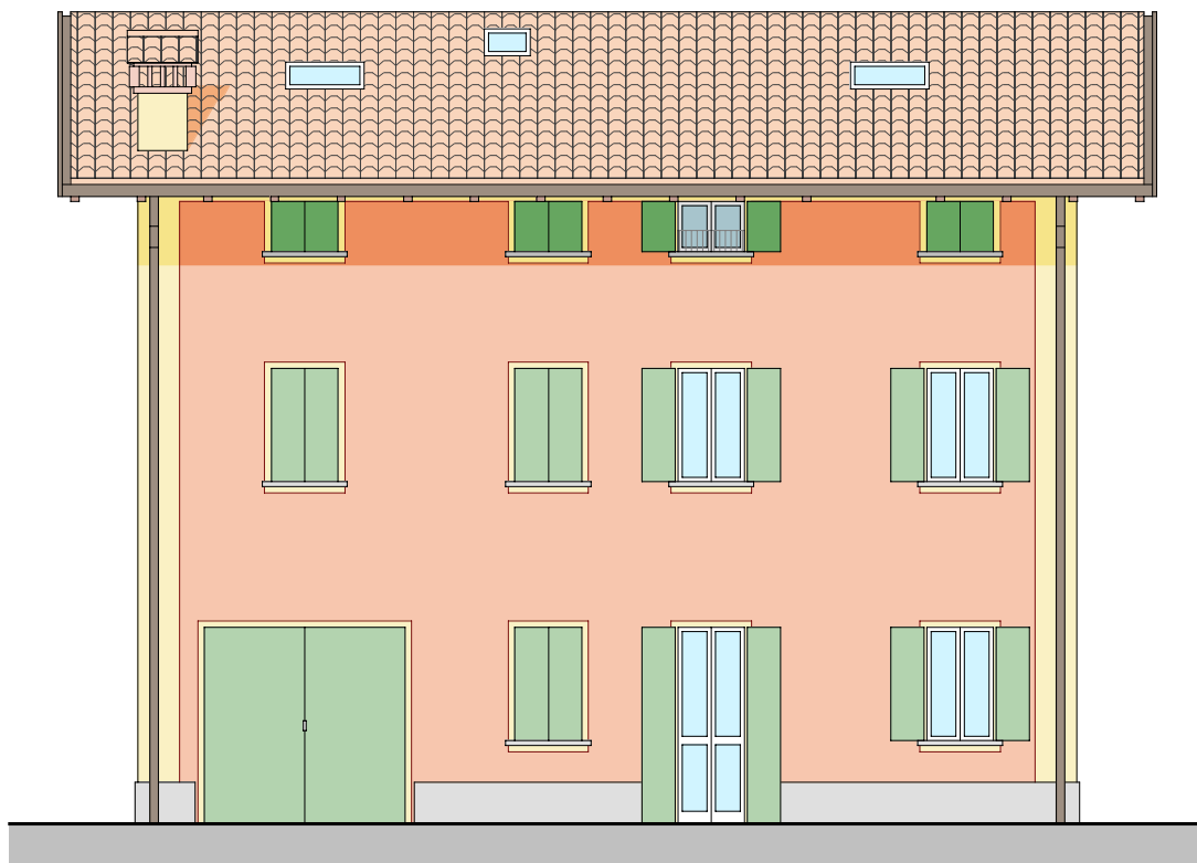
PROSPETTO SUD
