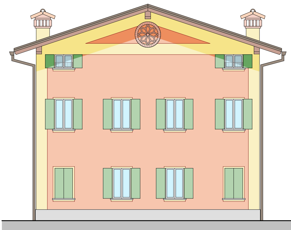
PROSPETTO OVEST
