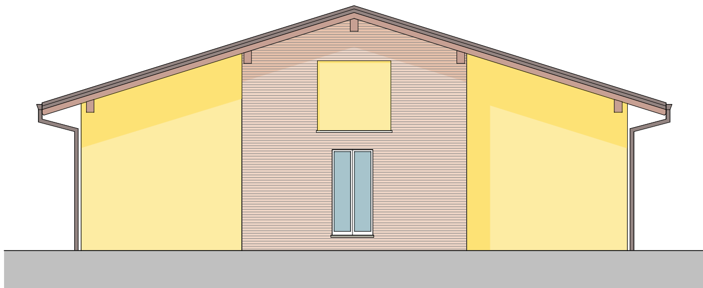
PROSPETTO NORD
