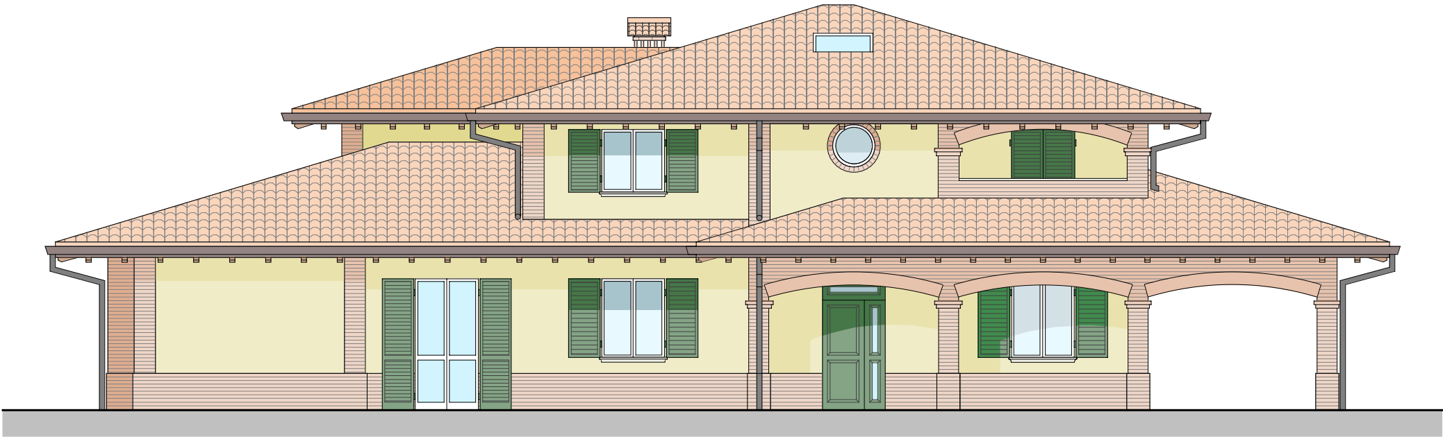
PROSPETTO NORD
