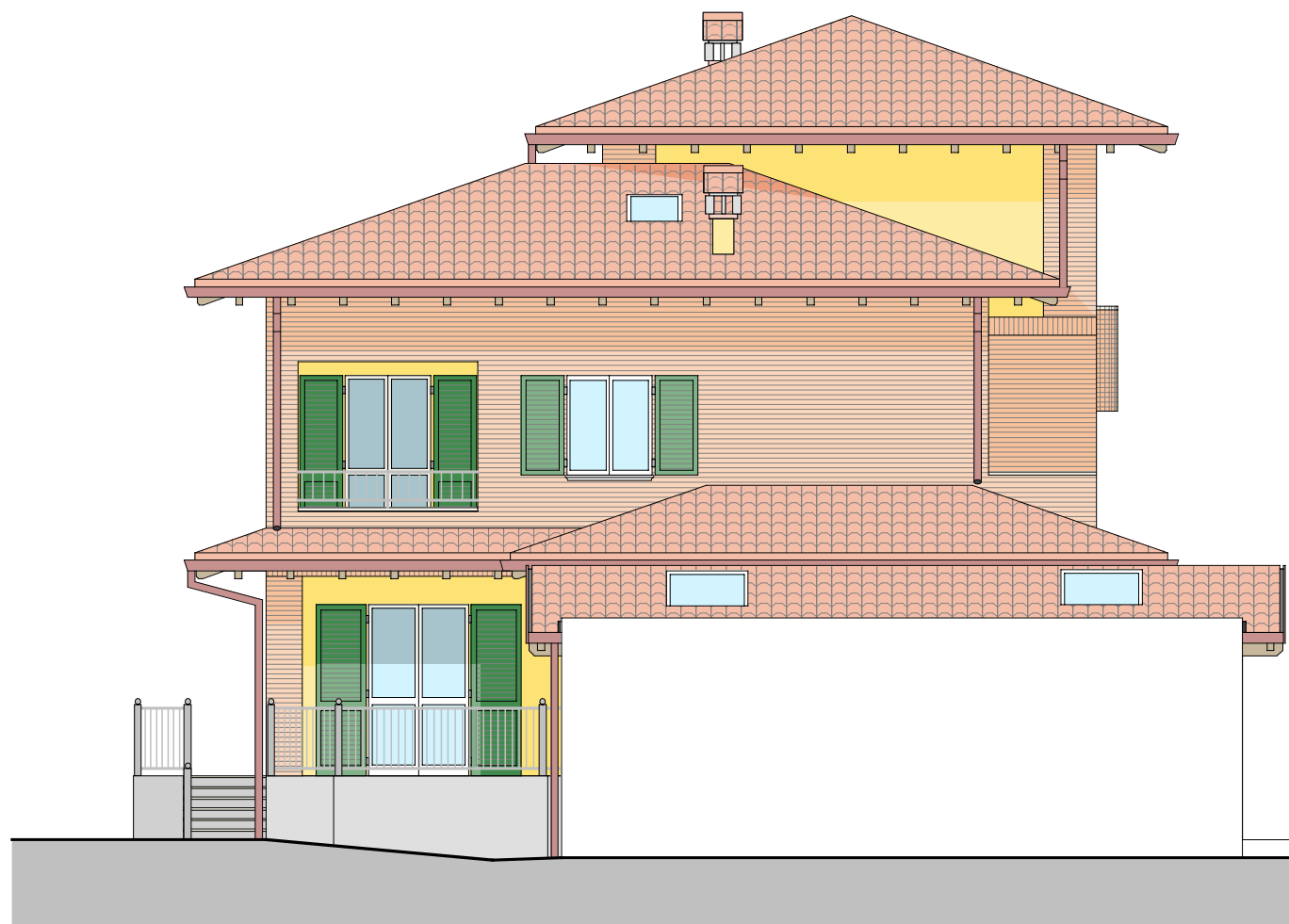
PROSPETTO EST
