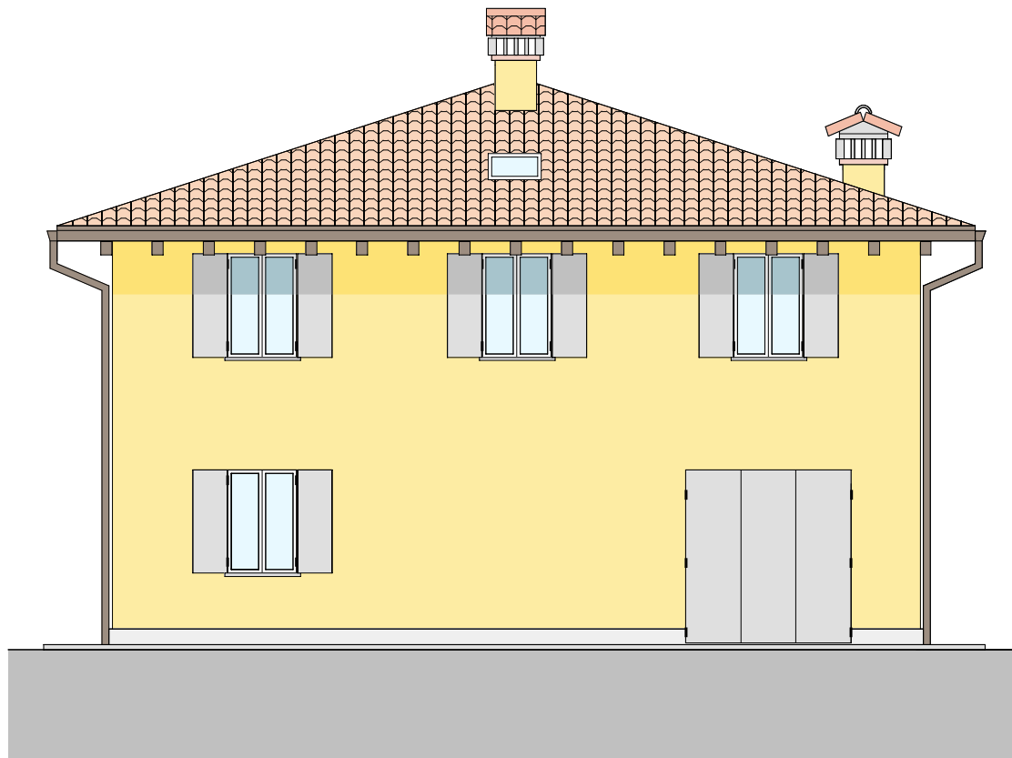
PROSPETTO NORD
