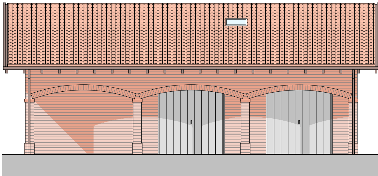
PROSPETTO OVEST
