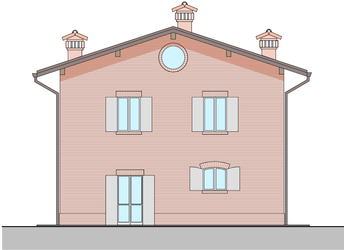
PROSPETTO OVEST
